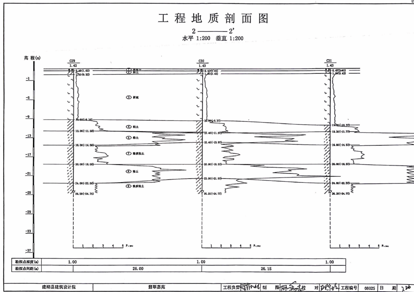
图 3.1-1 工程地质剖面图 (引自参考地勘)
