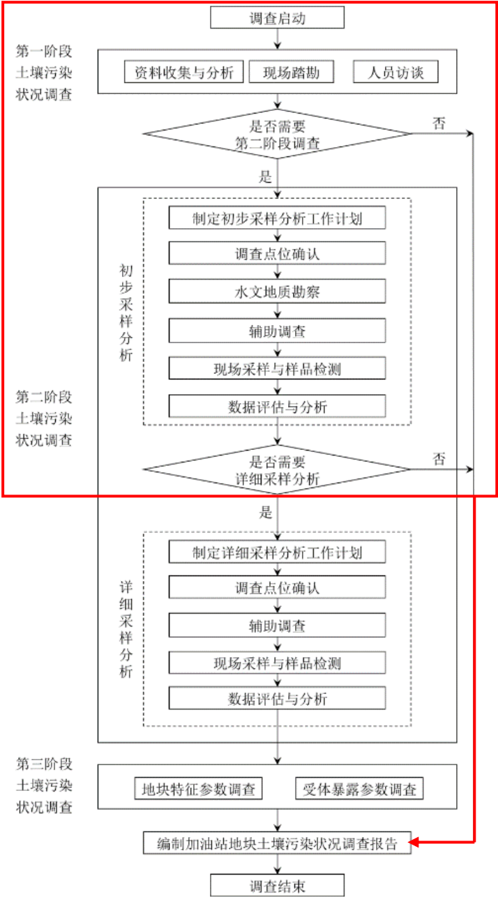
图 2.4-1 工作流程图
